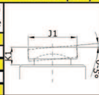
Dimensões do Assento Oscilante Opcional Montado com Parafuso (mm)
